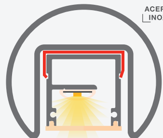
COMENZA Ø42.4x37mm
